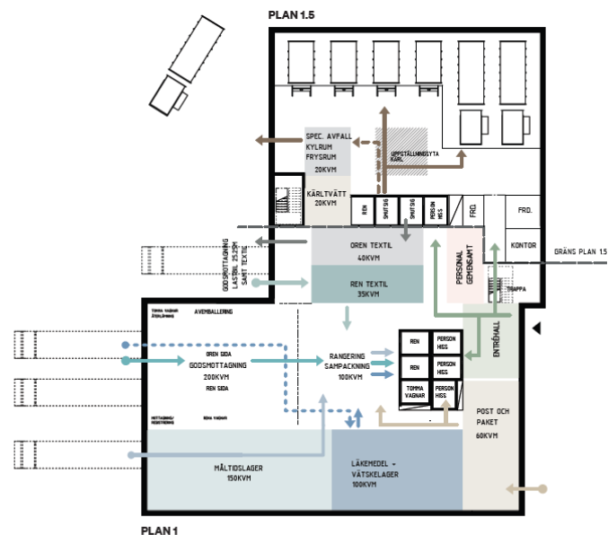
Skiss 23-08-22, servicebyggnad plan 09-10
