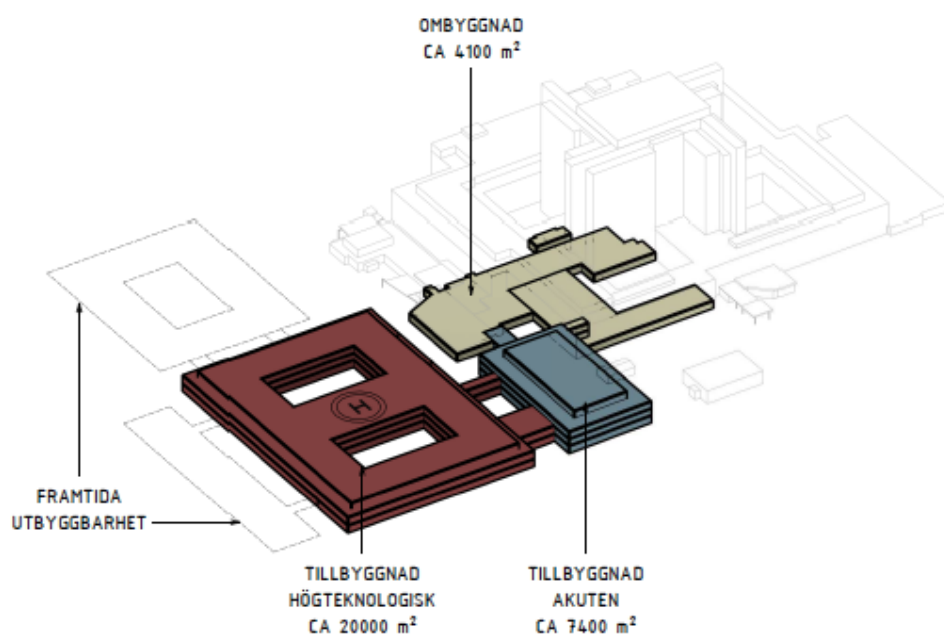
Skiss 23-08-28, situationsplan och volymsskiss
